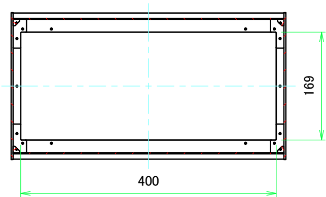
B-B ( 1 : 6 )
