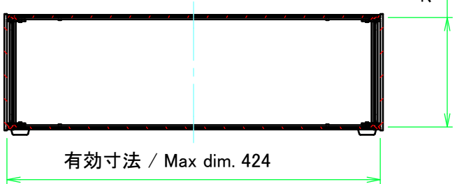
C-C ( 1 : 6 )
